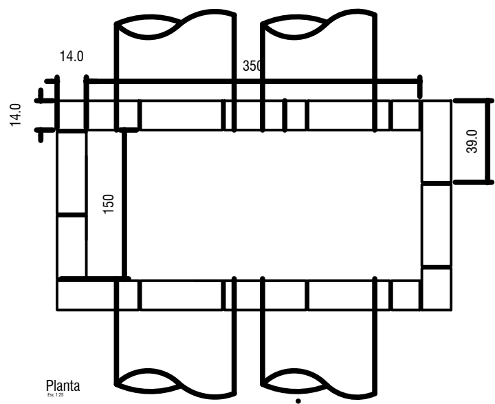
DETALHE / CAIXA DE LIGAÇÃO Escala 1:25
