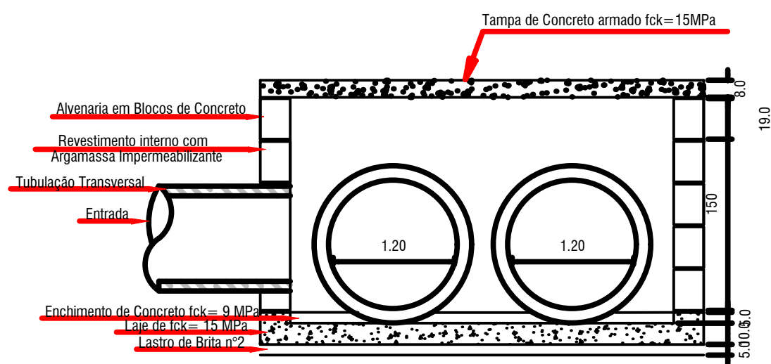
Corte Esc 1:25
