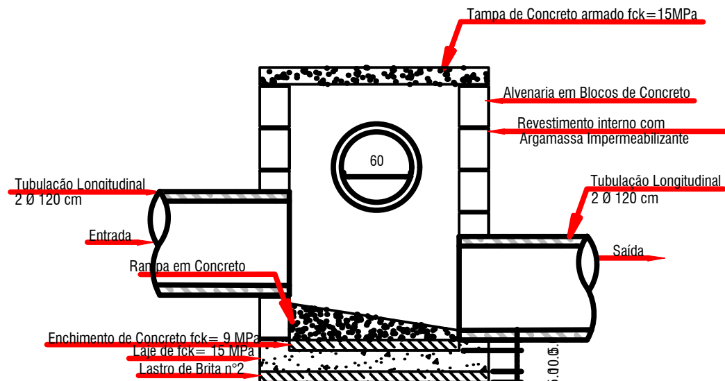
Corte Esc 1:25
