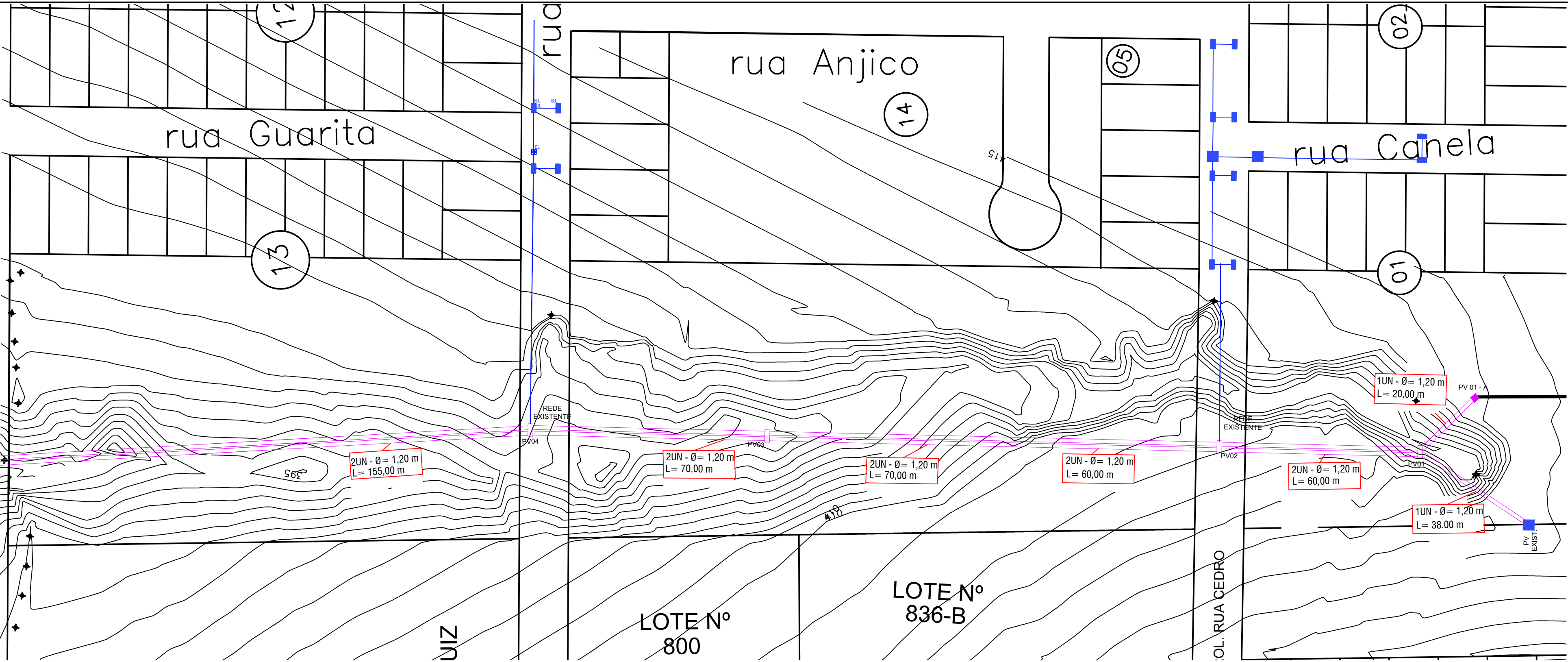
PLANTA BAIXA DRENAGEM Escala 1:1.500
