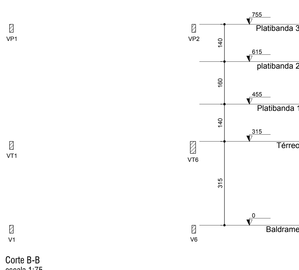
Corte B-B escala 1:75
